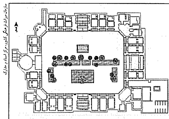
نقشه کف‌بنای مدرسه جدّه بزرگ
